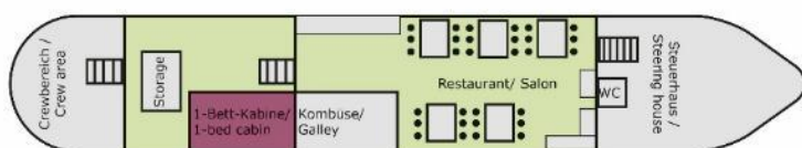
Hauptdeck / Main Deck
